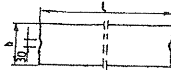
Rys. 1. Wymiarowanie krawężników
