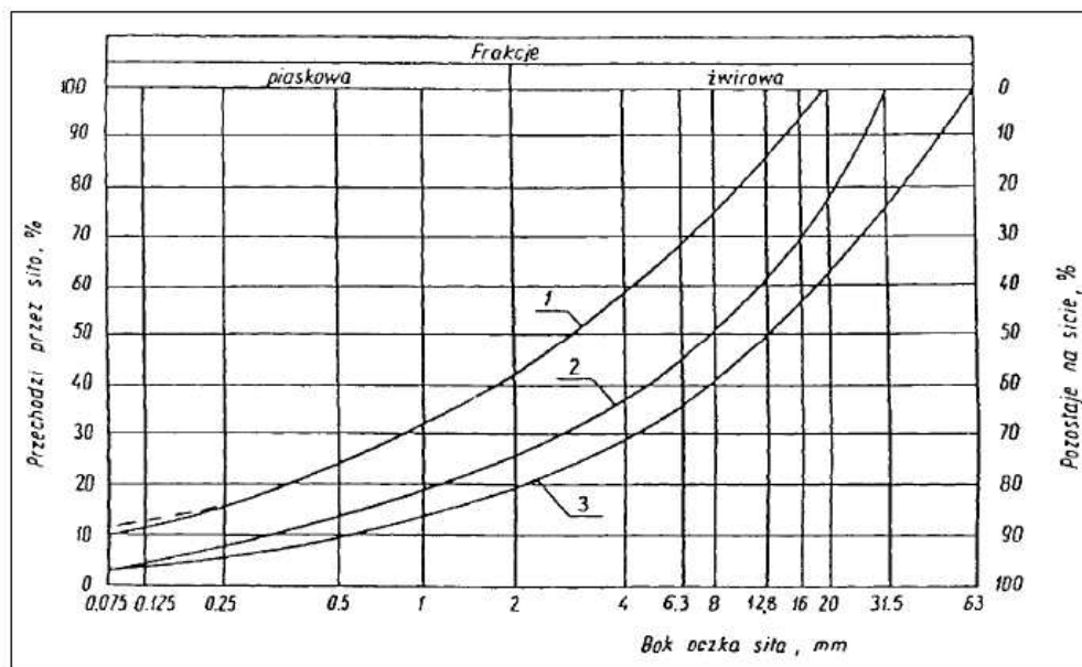
Rysunek 1 - Pole dobrego uziarnienia kruszyw przeznaczonych na podbudowy wykonywane metoda stabilizacji mechanicznej.
