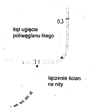
DETAL ŁĄCZENIA ŚCIAN
