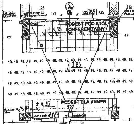
SALA KONFERENCJI. RZUT. SKALA 1:100.
