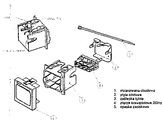
Rys.1. Uniwersalne ekranowane gniazdo teleinformatyczne skośne 2GHz Uniwersalne ekranowane złącze 8-pozycyjne 2GHz zostało zaprojektowane do współpracy z drutem miedzianym o średnicy 0,50 - 0,65mm (24 - 22 AWG), będącym elementem kabla
