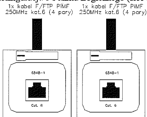
Rys. 3. Konfiguracja 2 Punktu Logicznego (sieć logiczna).
