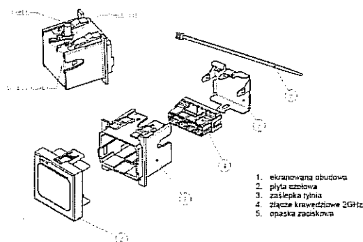
Rys.1. Uniwersalne ekranowane gniazdo teleinformatyczne skośne 2GHz Uniwersalne ekranowane złącze 8-pozycyjne 2GHz zostało zaprojektowane do współpracy z drutem miedzianym o średnicy 0,50 - 0,65mm (24 - 22 AWG), będącym elementem kabla 4-parowego podwójnie ekranowanego PiMF - S/FTP lub F/FTP o impedancji falowej 100 Ω. Proces
