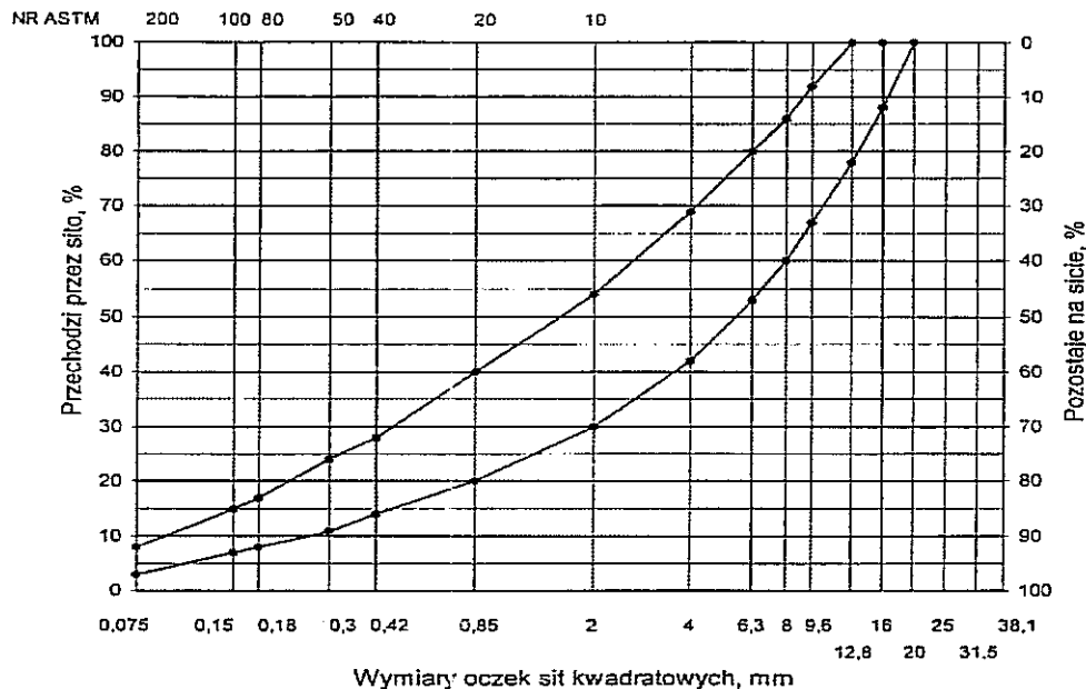
Rys. 9. Krzywe graniczne uziarnienia mieszanki mineralnej BA od 0 do 16 mm do warstwy wiążącej nawierzchni drogi o obciążeniu ruchem KR2
