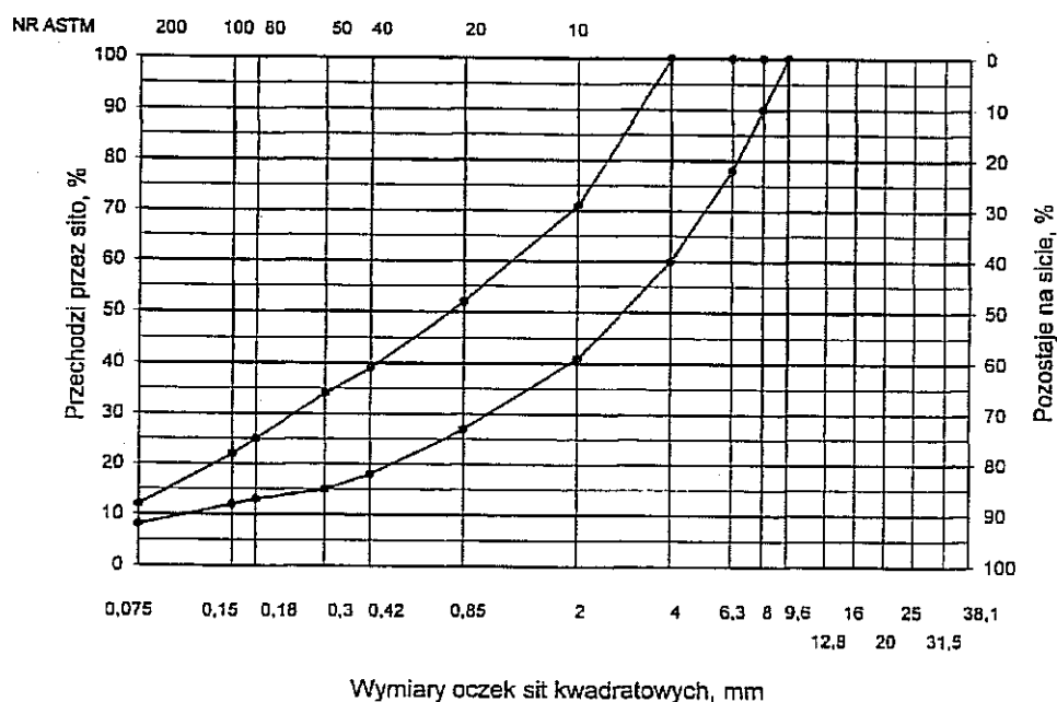
Rys. 3. Krzywe graniczne uziarnienia mieszanki mineralnej BA od 0 do 8mm, do warstwy ścieralnej nawierzchni drogi o obciążeniu ruchem nawierzchni drogi o obciążeniu ruchem KR2
