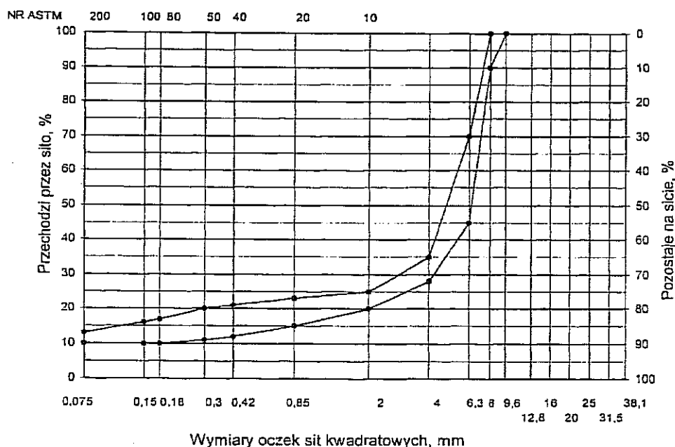
Rys. 7. Krzywe graniczne uziarnienia mieszanki mineralnej SMA od 0 do 8 mm do warstwy ścieralnej nawierzchni drogi o obciążeniu ruchem KR3
