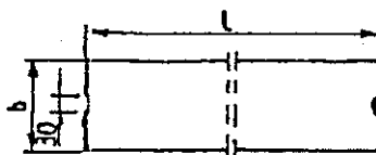
Rys. 1. Wymiarowanie krawężników
