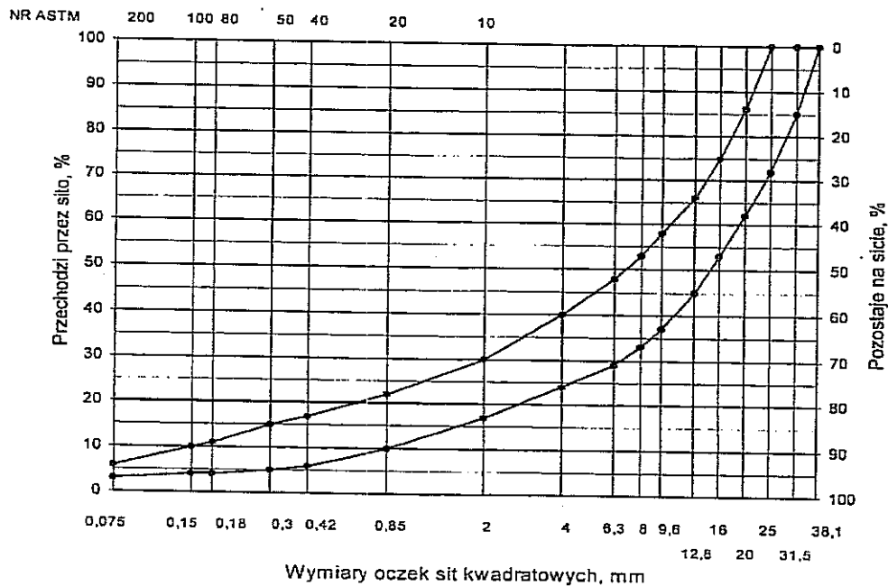
Rys. 6. Krzywe graniczne uziarnienia mieszanki mineralnej BA od 0 do 31,5 mm podbudowy nawierzchni drogi o obciążeniu ruchem od KR 3 do KR 5
