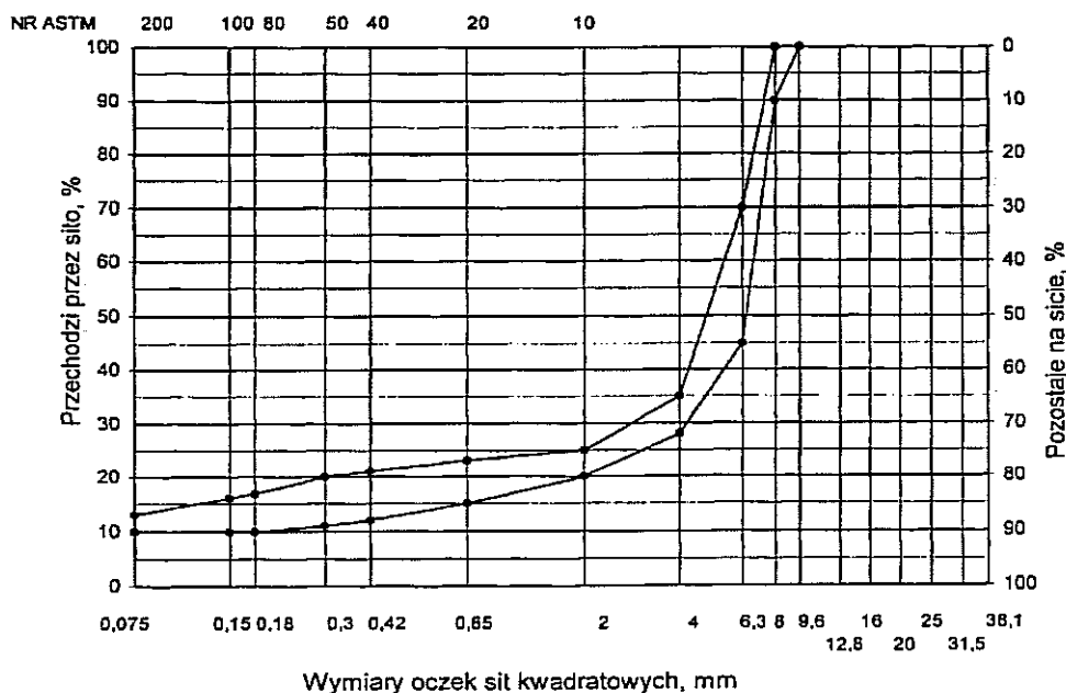
Rys. 1. Krzywe graniczne uziarnienia mieszanki mineralnej SMA od 0 do 8 mm do warstwy ścieralnej nawierzchni drogi o obciążeniu ruchem od KR3 do KR6
