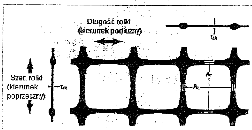
Rys. 1. Struktura georusztu
