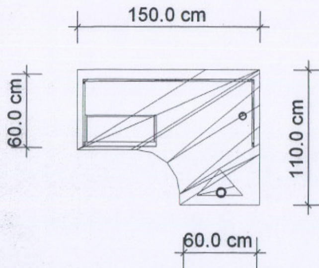
Biurko kształtowe pod komputer-"lewe" 1500/1100/600/760 szer./gł./wys. [mm]
