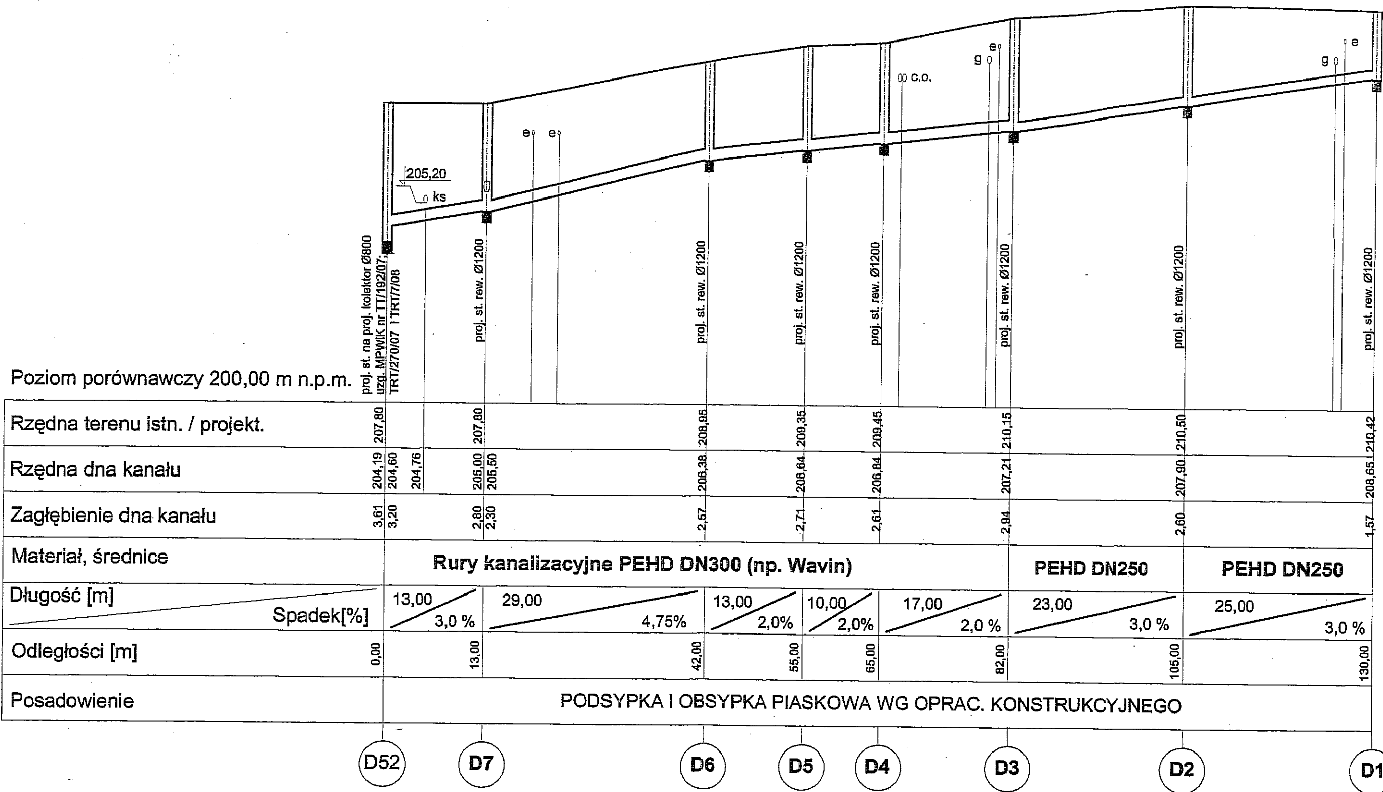
PROFIL PODŁUŻNY SIECI KANALIZACJI DESZCZOWEJ 1:100/500
