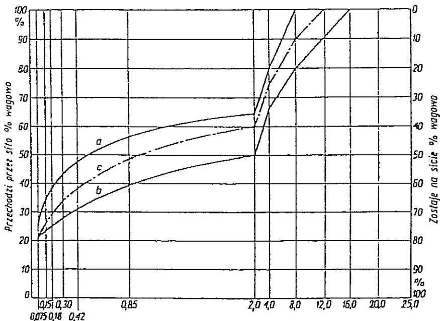
Rys. 1. Krzywe graniczne uziarnienia mieszanki mineralnej dla średnioziarnistej mieszanki asfaltu lanego:
