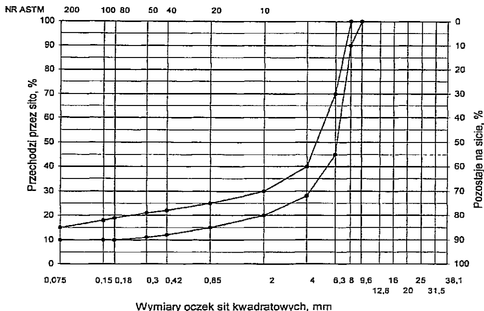
Rys. 1. Krzywe graniczne uziarnienia mieszanki mineralnej SMA od 0 do 8 mm do warstwy ściernalnej nawierzchni drogi o obciążeniu ruchem KR2
