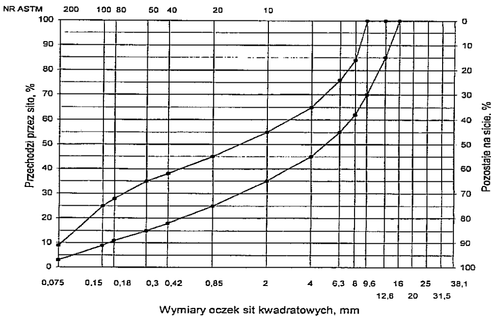
Rys. 1. Krzywe graniczne uziarnienia mieszanki mineralnej BA od 0 do 12,8 mm do warstwy wyrównawczej nawierzchni drogi o obciążeniu ruchem KR2
