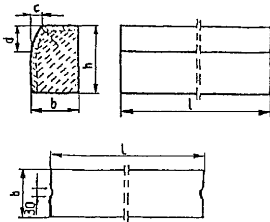
Rys. 1. Wymiarowanie krawężników
