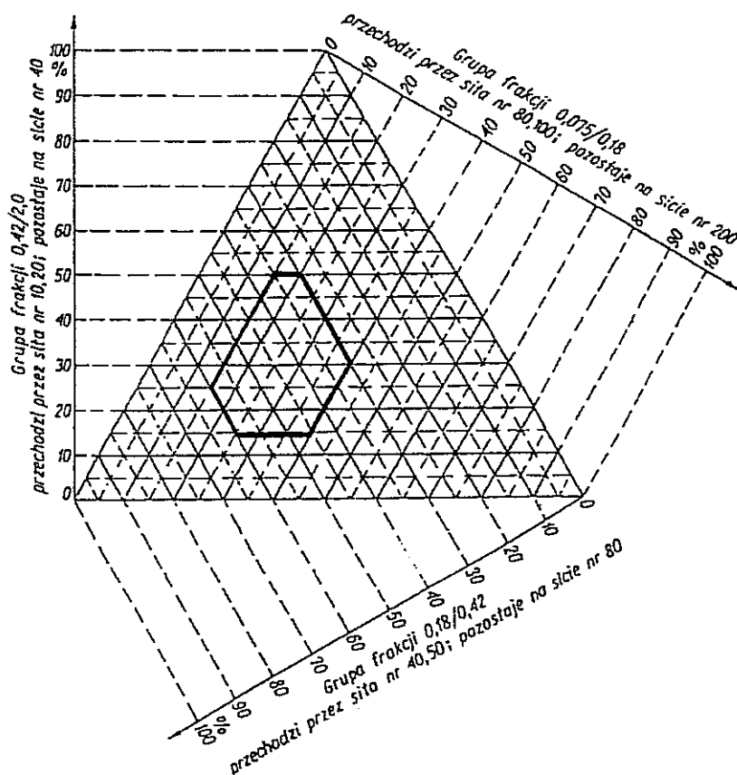
Rys. 1. Krzywe graniczne uziarnienia mieszanki mineralnej dla średnioziarnistej mieszanki asfaltu lanego: a, b - dla dróg międzymiastowych; b, c - dla dróg miejskich, mostów.
