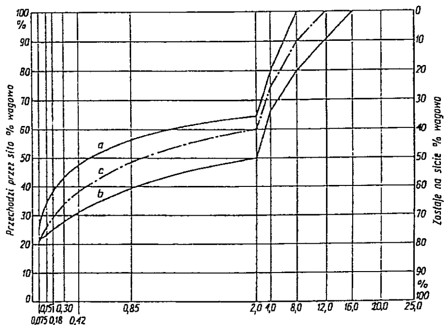
Rys. 1. Krzywe graniczne uziarnienia mieszanki mineralnej dla średnioziarnistej mieszanki asfaltu lanego: a, b - dla dróg międzymiastowych; b, c - dla dróg miejskich, mostów.
