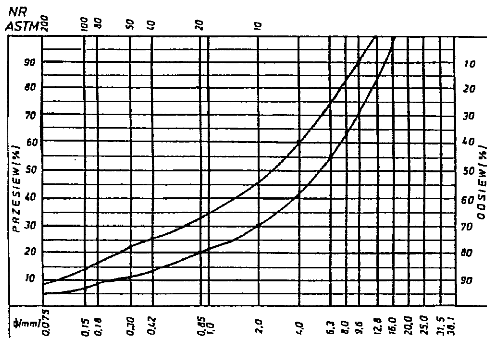
Rys. 13. Krzywe graniczne uziarnienia mieszanki mineralnej 0÷16 mm do warstwy wiążącej, z betonu asfaltowego dla KR 3
