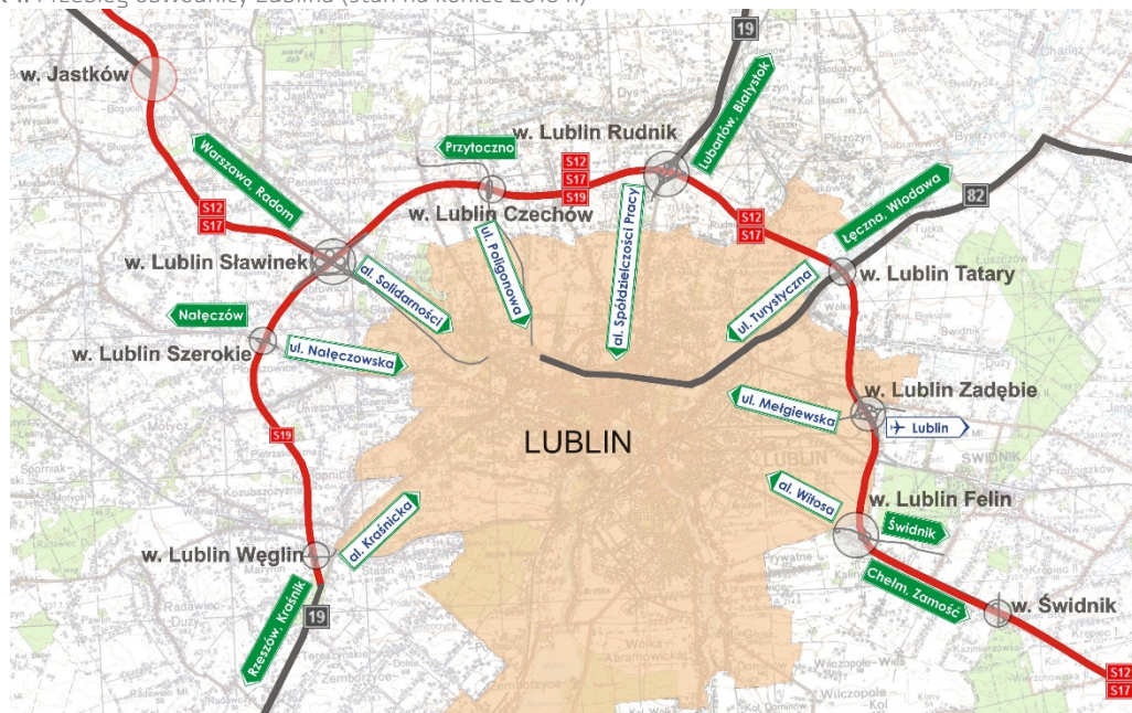
Rysunek 1. Przebieg obwodnicy Lublina (stan na koniec 2016 r.)
